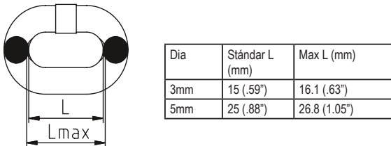
Cadena de mano - longitud de un enlace
