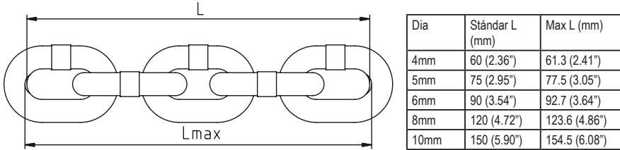
Cadena de carga - longitud de cinco eslabones
